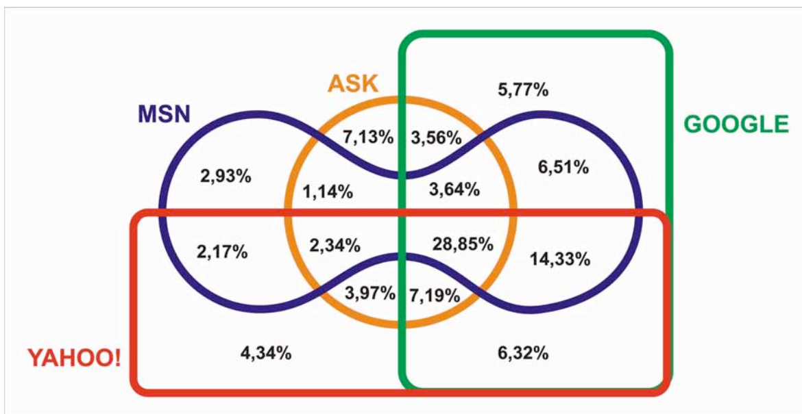
Figura 4: Representação gráfica das porcentagens da web indexável nos bancos de dados dos maiores buscadores. REPRODUZIDO DE GULLI E SIGNORINI, 2005, p. 2.
